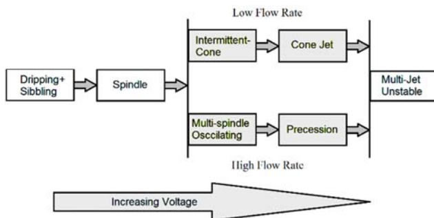
Fig. 19 Flow chart of spray mode in electric field شکل 19 چارت تغییرات حالت‌های الکترواسپری داخل میدان الکتریکی
