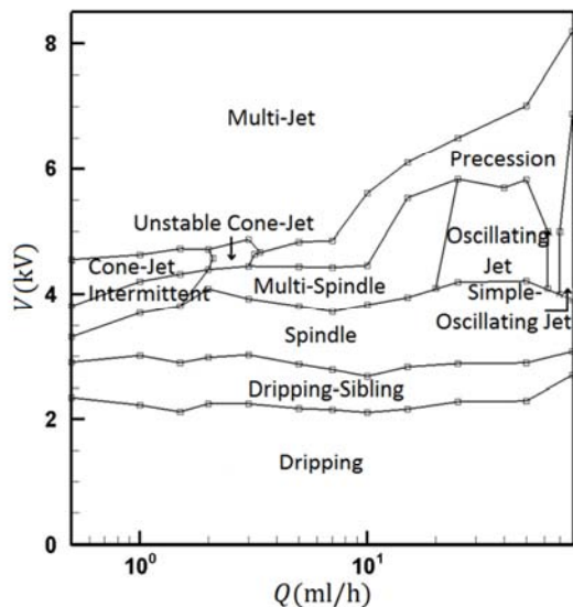
Fig. 18 The operating ranges of different spraying modes for ethanol شکل 18 دامنه‌ی عملیاتی مدهای مختلف الکترواسپری برای اتانول
