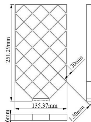
Fig. 14 The Grid fin model
