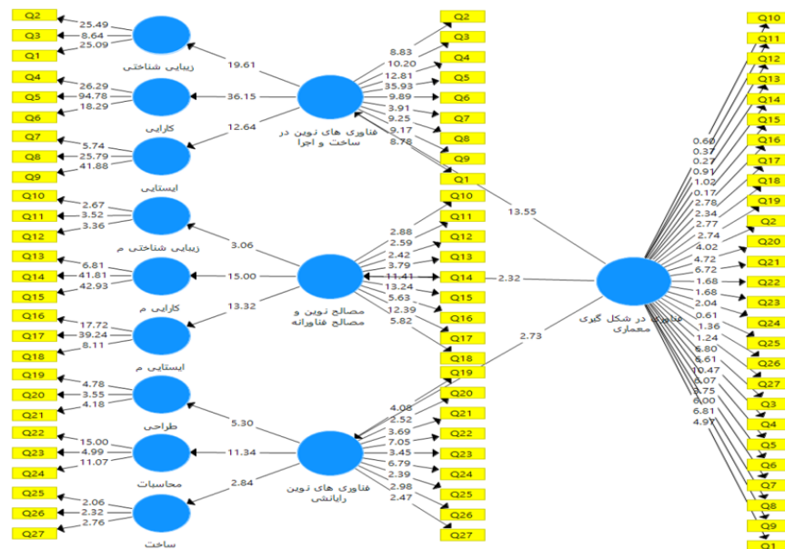
شکل - ۲: ضرایب معناداری آزمون t مدل اندازه‌گیری
