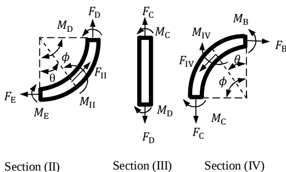
Fig. 6 Forces and momentum for different regions of sheet شکل 6 نیروها و گشتاور در نواحی مختلف ورق
