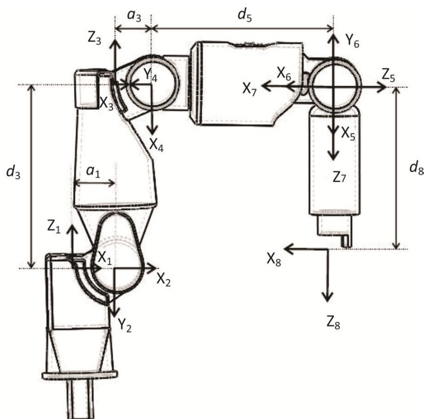
شکل 2 شکل دو بعدی بازوی رباتیکی به همراه ابعاد اصلی a_1, a_3, a_5, a_7, d_3, d_5, d_7, d_8
