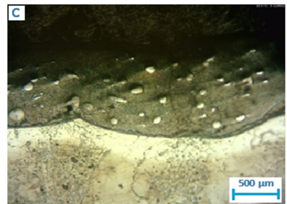
شکل 13 اثر هم‌پوشانی پاس‌ها (a: 30%, b: 50% و c: 70% هم‌پوشانی)
