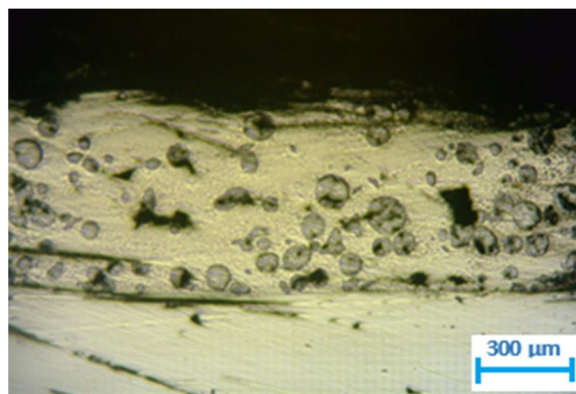
شکل 2 سطح مقطع پوشش با قدرت لیزر 167 وات، سرعت 5 میلی‌متر بر ثانیه و ارتفاع نقطه کانونی 5 میلی‌متر از سطح قطعه
