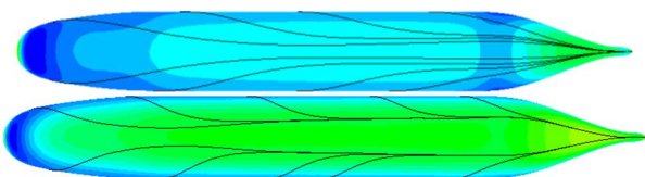
شکل 10 خطوط تنش برشی بر روی بدنه زیرسطحی سابوف در زوایای حمله مختلف (زاویه حمله 15 درجه (بالا) و زاویه حمله 30 درجه (پایین))
