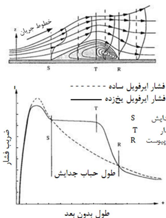
شکل 1 تحلیل میدان جریان و توزیع فشار برای حباب جدایش آرام لبه حمله بر روی ایرفویل یخ زده [6]
