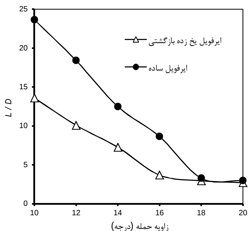
شکل 22 تغییرات نسبت آیرودینامیکی برآ به پسا بر حسب زاویه حمله برای ایرفویل NACA23012
