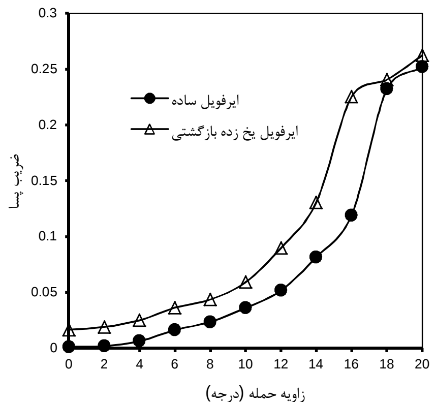
شکل 21 تغییرات ضریب پسا بر حسب زاویه حمله برای ایرفویل NACA23012
