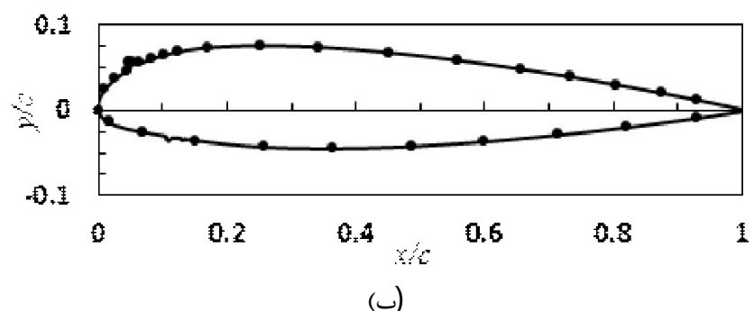
شکل 5 مختصات حفره های فشار برای ایرفویل بدون یخ (شکل الف) و ایرفویل یخزده NACA23012 (شکل ب)
