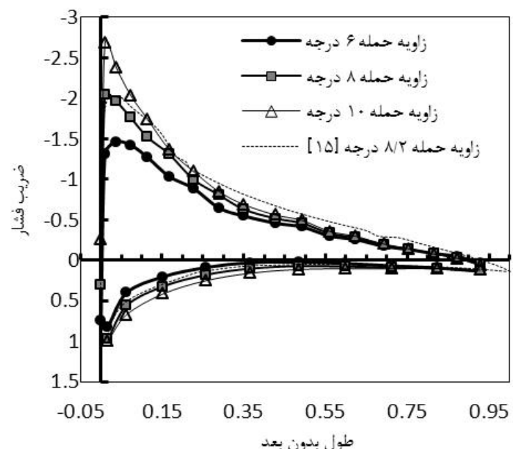
شکل 9 ضریب فشار بر حسب x/c در زوایای حمله 6، 8 و 10 درجه برای ایرفویل بدون یخ NACA 23012
