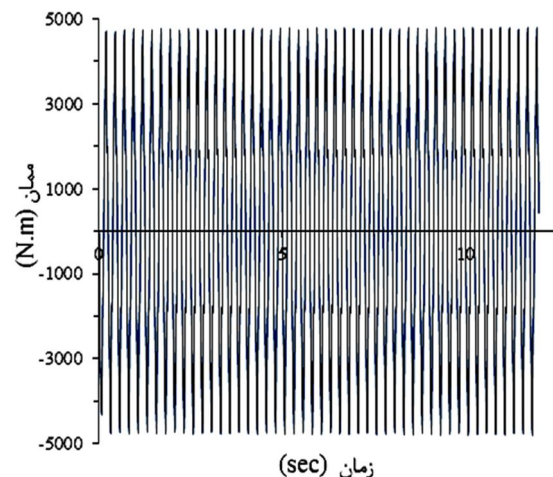
شکل 5 ممان به دست آمده از روش عددی
