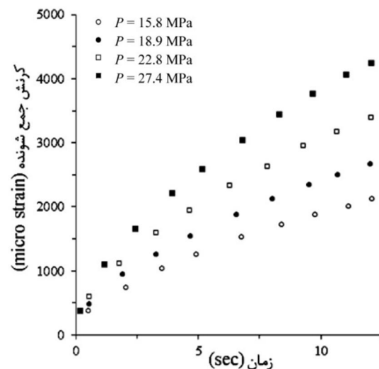
شکل 8 مقایسه کرنش‌های جمع شونده لوله زانویی از جنس فولاد ضدزنگ در فشارهای مختلف در فرکانس 4/00 هرتز
