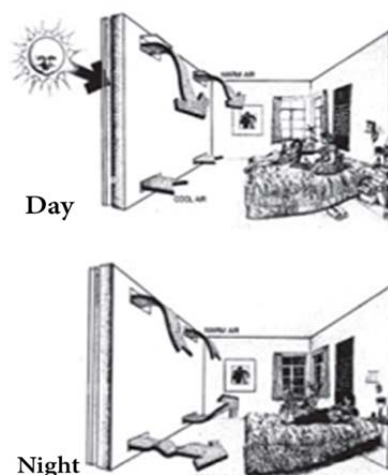
شکل ۶) عملکرد شبانه‌روز دیوار آبی [2]
