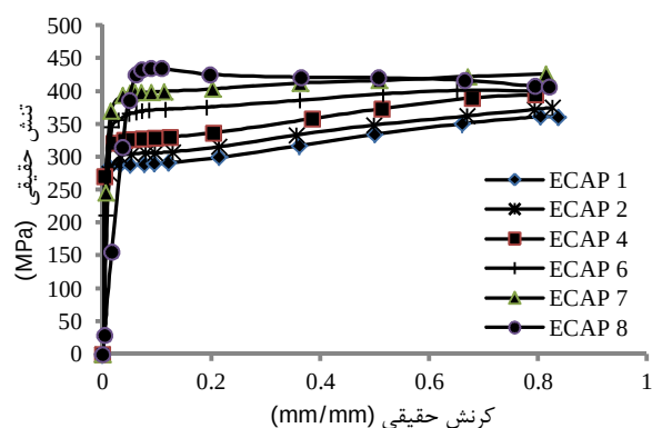
شکل 16 منحنی‌های تنش-کرنش فشاری مس تولید شده در پاس‌های 1، 2، 4، 6، 7 و 8 توسط قالب \phi = 110^\circ
