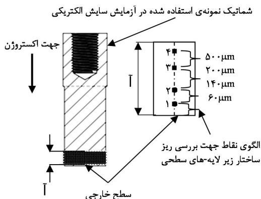
شکل 13 شماتیک برش طولی نمونه‌ی مورد استفاده برای آزمایش سایش الکتریکی به همراه الگوی نقاط بررسی زیر لایه‌های سطحی
