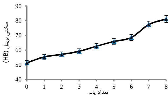
شکل 15 تغییرات سختی نمونه‌های مسی تولید شده در قالب \phi = 110^\circ به ازای هر مرحله اکستروژن
