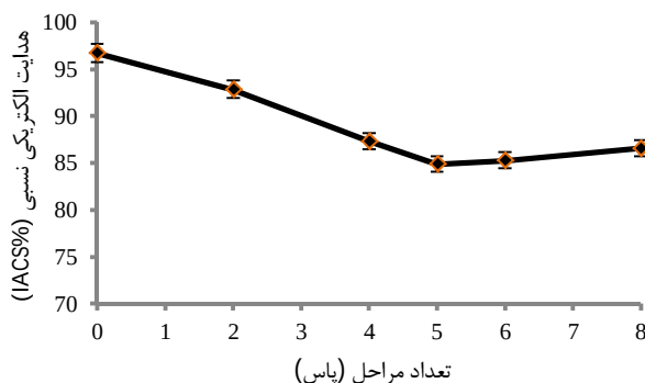
شکل 9 تغییرات هدایت الکتریکی نسبی بر حسب مراحل اکستروژن
