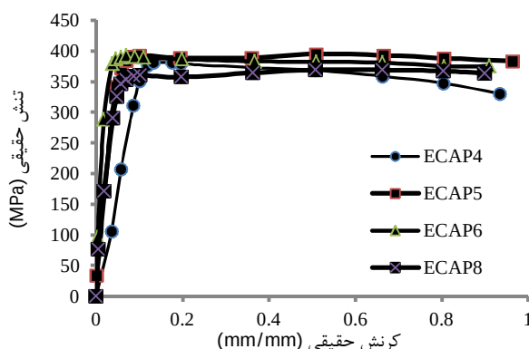
شکل 7 منحنی‌های تنش-کرنش فشاری مس پس از چهار تا هشت مرحله اعمال فرآیند ECAP
