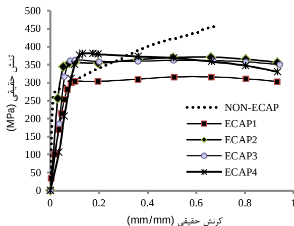
شکل 6 منحنی‌های تنش-کرنش فشاری مس پس از یک تا چهار مرحله اعمال فرآیند ECAP به همراه نمونه اولیه
