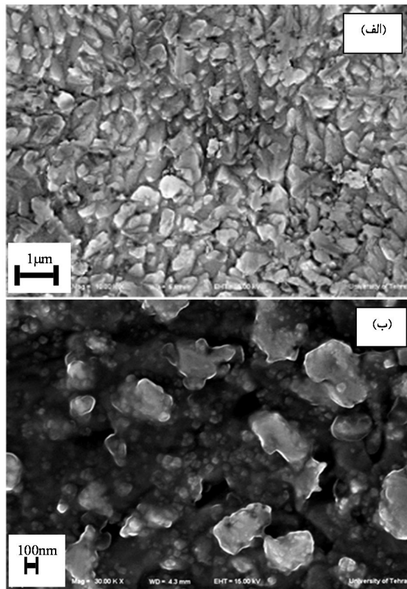
شکل 18 تصویر FE-SEM از ریز ساختار مس تولید شده توسط قالب \theta = 110^\circ در (الف) پاس 4 و (ب) پاس 8
