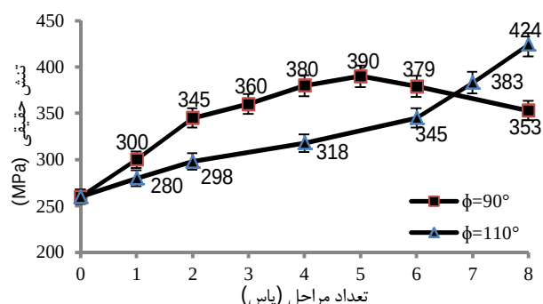
شکل 17 تغییرات تنش تسلیم مس تولید شده توسط دو قالب \phi = 90^\circ و \phi = 110^\circ بر حسب مراحل اکستروژن
