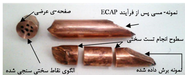
شکل 1 نمونه‌های ECAP شده و الگوی نقاط سختی سنجی
