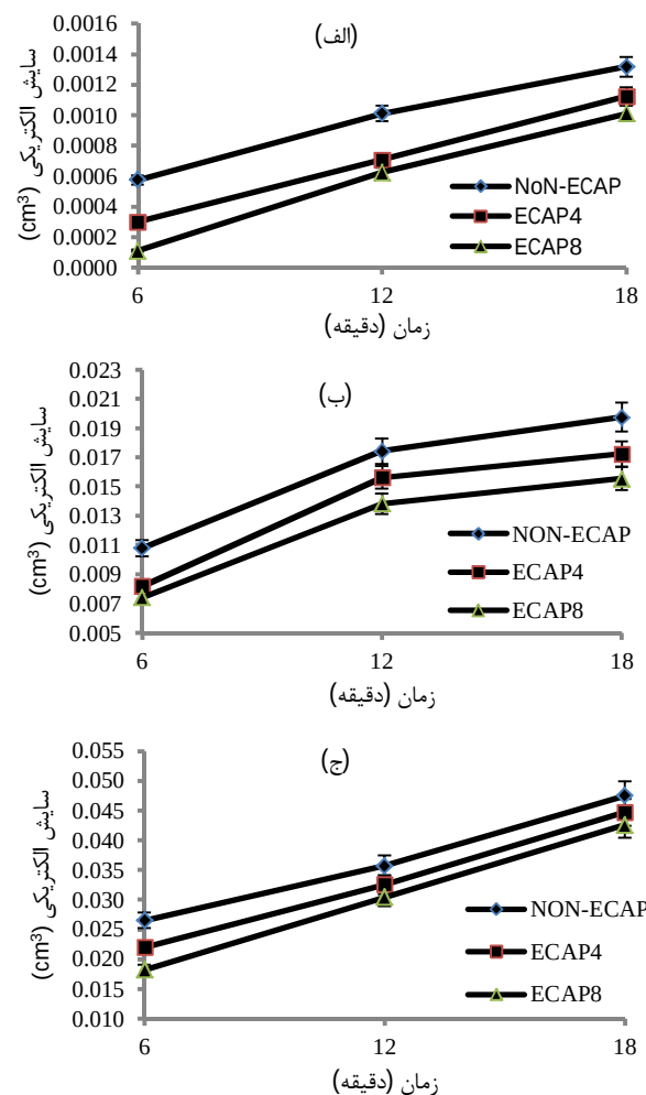
شکل 11 سایش الکتریکی نمونه‌های مسی ECAP4، ECAP8 و نمونه‌ی اولیه بر حسب زمان به ترتیب در شدت جریان‌های - الف) 5 ب) 10 و ج) 15 آمپر
