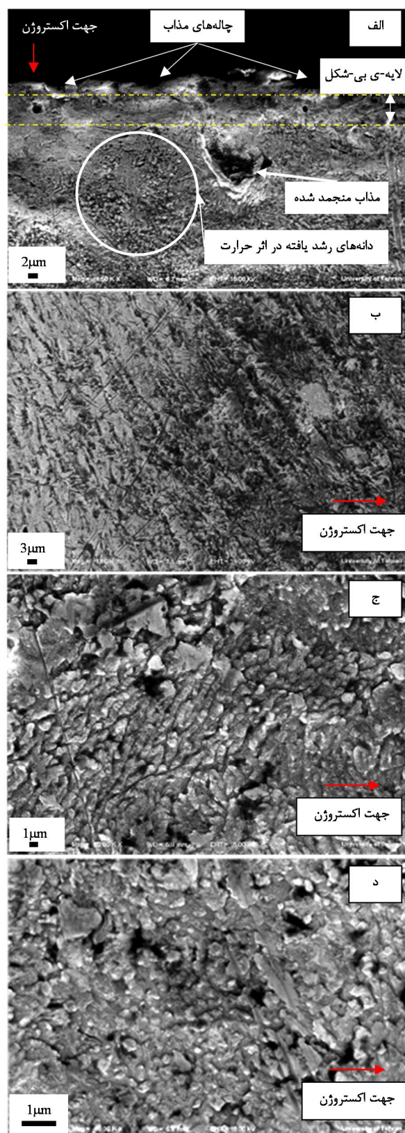
شکل 14 تصویر FE-SEM از ریز ساختار زیر لایه‌ی عمق - الف) 60 \mu\text{m} (ب) 200 \mu\text{m} (ج) 400 \mu\text{m} (د) 900 \mu\text{m}
