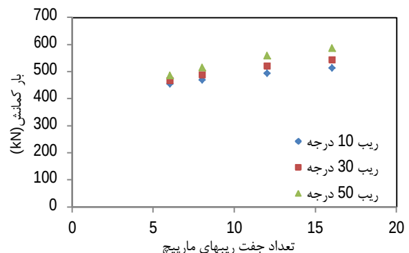
شکل 15 نمودار تغییرات بار کمانش بر حسب تعداد جفت ریبهای مارپیچ به ازای زوایای مختلف ریب مارپیچ
