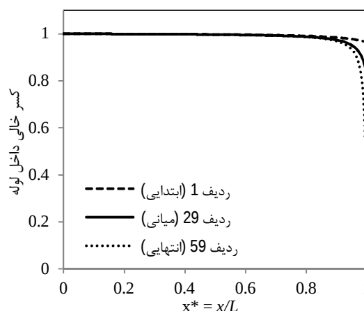
شکل 11 نمودار تغییرات کسر خالی داخل لوله در طول لوله
