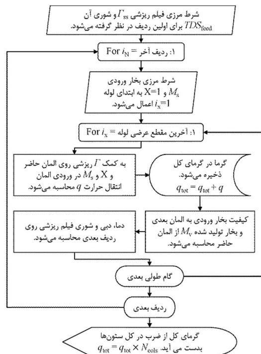
شکل 5 فلوجارت الگوریتم ارائه شده جهت شبیه‌سازی تبخیر فیلم ریزشی روی ردیف‌های دسته‌لوله.
