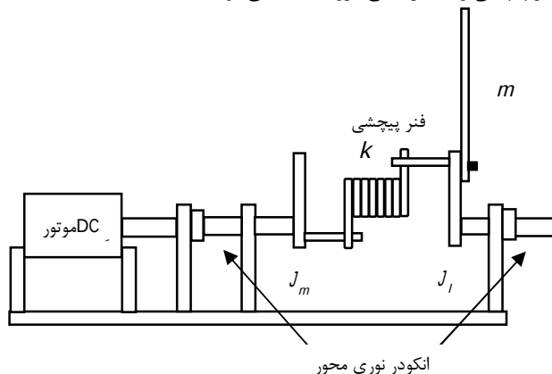
شکل 1 طرح ربات تک بازو با مفصل انعطاف پذیر [23]
