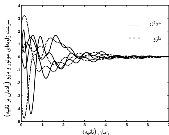
شکل 11 توافق جمعی در سرعت زاویه‌ای موتور و بازو، کنترل گر مرتبه‌ی شش
