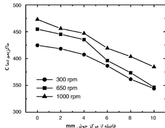
شکل 2 تأثیر سرعت دورانی بر روی بیشینه دما
