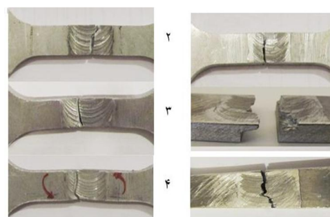
شکل 16 نواحی بروز شکست در نمونه
