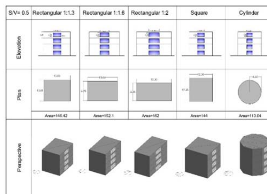
شکل ۱) احجام ساده مدل سازی شده
