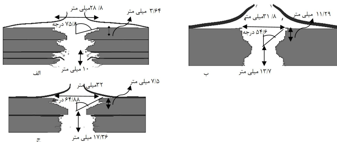
شکل ۹ مشخصات هندسی عمق، زاویه، طول و ارتفاع پای شکست مخروطی در زره سرامیکی الف) 2(E(0.5)C(4))2(E(0.5)C(8))2 (ب) E(2)C(25) ج) 2(E(1)C(12))2
