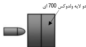
اجزای مدل هدف ولدوکس 700 ای روکش هسته فیلمر جلویی فیلمر عقبی تعداد المان 2400 828 1068 1526 تعداد گره 2562 978 1167 1660
