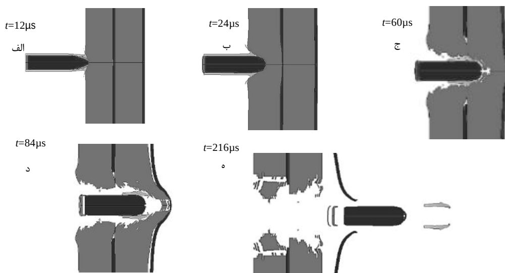
شکل 7 مکانیزم نفوذ گلوله ضد زره روکش‌دار در هدف سرامیکی دو لایه 2(C12)(E1)
