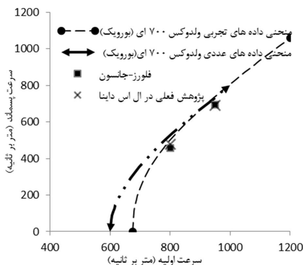
شکل 5 منحنی و داده‌های سرعت اولیه-سرعت پسماند برای هدف "دی 12 دلیو" [۲، ۱]
