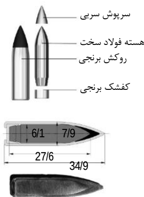
شکل 1 طرح و هندسه گلوله "ای پی ام 2" کالیبر 7/62 [1]
