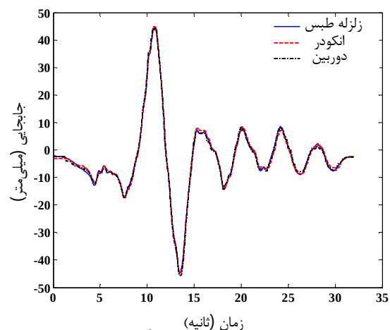
شکل 11 مقایسه بین ورودی مرجع (زلزله‌ی طبس) و جابجایی اندازه‌گیری شده توسط انکودر و برنامه‌ی پردازش تصویر (بازخورد دوربین)
