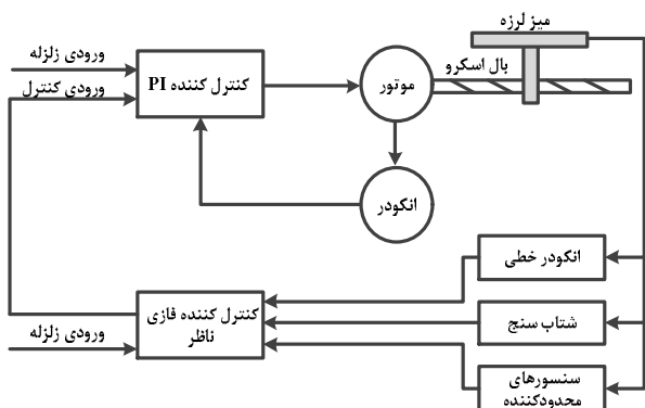
شکل 2 ساختار کنترلی میز لرزه
