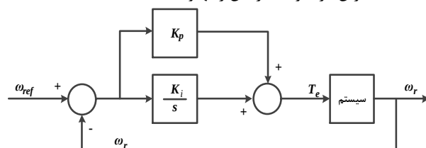
شکل 3 ساختار کنترل کننده‌ی تناسبی- انتگرال گیر
