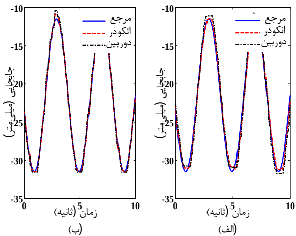
شکل 10 مقایسه‌ی بین مقدار مرجع و جابجایی اندازه‌گیری شده توسط انکودر و دوربین در حالت آنلاین (الف) سیستم قبلی با بازخورد انکودر (ب) سیستم پیشنهادی با بازخورد دوربین
