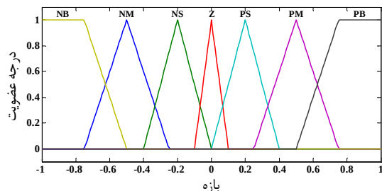
شکل 6 توابع تعلق مربوط به ورودی خطای جابجایی و مشتق آن
