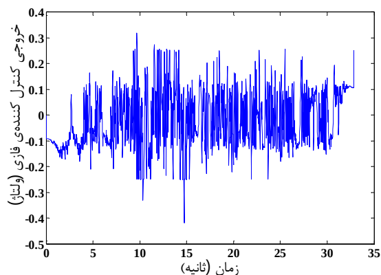
شکل 12 تغییرات خروجی کنترل کننده فازی در شبیه‌سازی زلزله‌ی طبس
