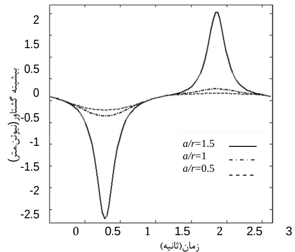
شکل 11 گشتاور ساختار در نسبت‌های هندسی گوناگون
