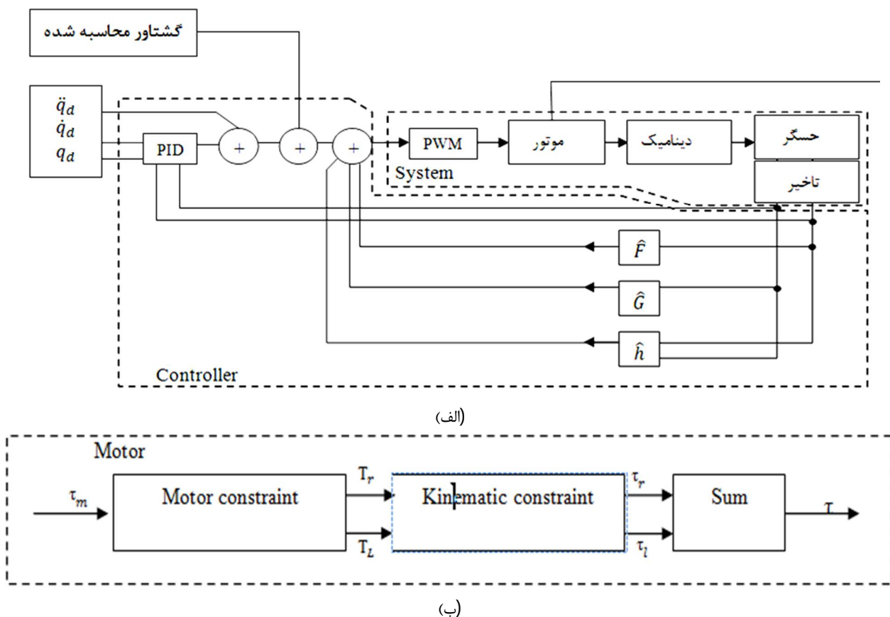
شکل 4 (الف) فلوچارت کنترلی (ب) ساختار موتور در الگوریتم حل مسئله
