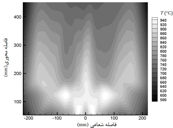
شکل ۱۷ توزیع دما در L=3R و \phi = 0.68
