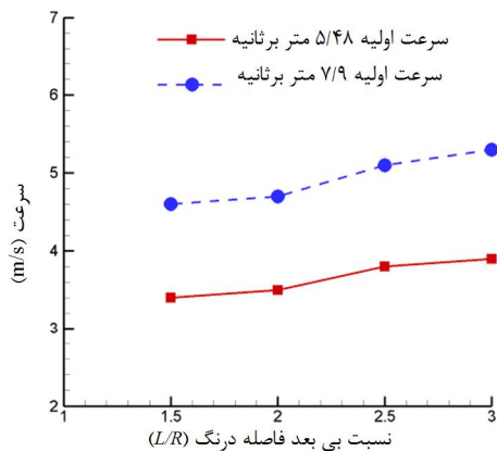
شکل ۹ میانگین سرعت اندازه‌گیری شده بر روی سر مشعل در حالت سرد (غیر واکنشی) و با تغییر میزان فاصله درنگ در دو سرعت اولیه
