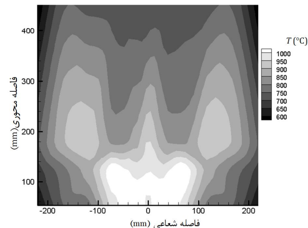
شکل ۱۸ توزیع دما در L=3R و \phi = 0.78
