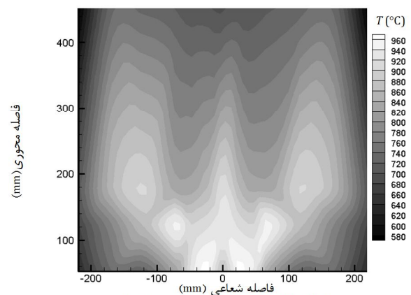
شکل ۱۵ توزیع دما در L=2R و \phi = 0.68
