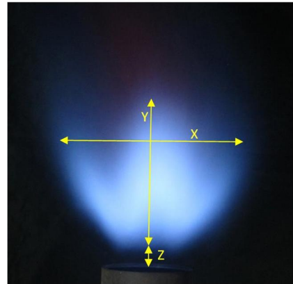
شکل ۷ تصویر شعله برخاسته مشعل کم‌پیچش و پارامترهای قابل اندازه‌گیری
