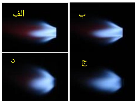
شکل ۱۹ تصاویر شعله کم‌پیچش (چسبیده و برخاسته) در یک هندسه و فاصله درنگ
