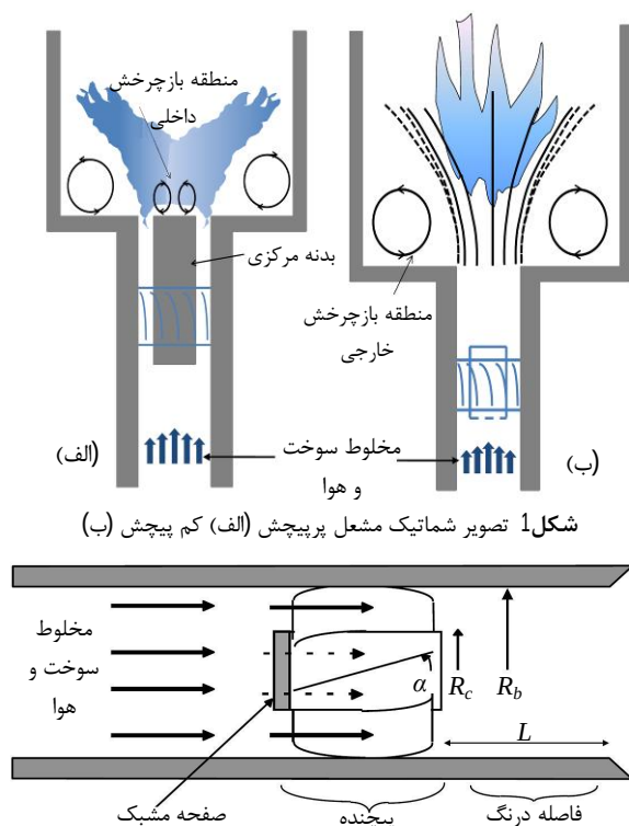
شکل 1 تصویر شماتیک مشعل پرپیچش (الف) کم پیچش (ب)
