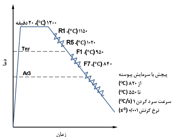
شکل 4 چرخه ترمومکانیکی انجام آزمون پپچش گرم با زمان بندی واقعی به همراه پپچش با سرمایش ییوسته.
