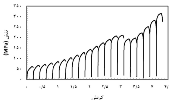
شکل 5 نمودارهای تنش-کرنش حاصل از آزمون پیچش گرم با زمان بندی میانگین.
