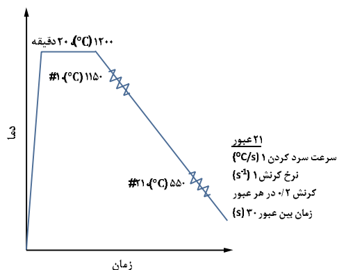
شکل 3 چرخه ترمومکانیکی رایج انجام آزمون پیچش گرم با زمان بندی میانگین برای تعیین دماهای بحرانی [10-13].
