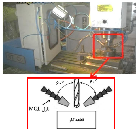
شکل 4 چیدمان انجام آزمایش به همراه دستگاه MQL استفاده‌شده
