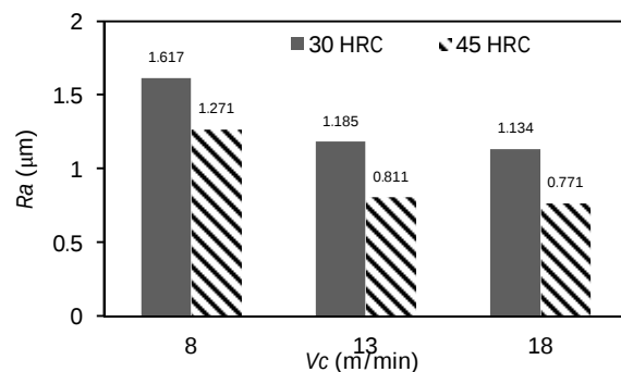
شکل 13 تأثیر تغییرات سرعت برشی بر زبری سطح سوراخ
