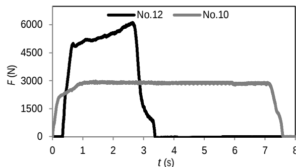
شکل 7 مقایسه نیروی برشی در آزمایش‌های 10 و 12
