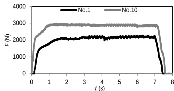
شکل 11 مقایسه نیروی برشی در آزمایش‌های 1 و 10
