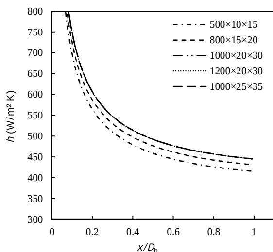
شکل 2 بررسی استقلال حل از شبکه برای h با Gr = 5 \times 10^5 ، Q_r = 1 ، Re = 700 و AR = 0.5 ، \phi = 1\%
