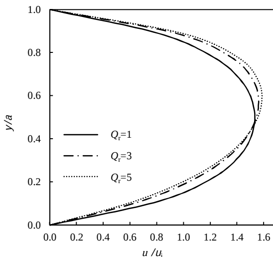
شکل 10 پروفیل سرعت بی بعد در مقطع x/D_h = 50 برای مقادیر مختلف Q_f
