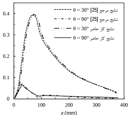
شکل 4 مقایسه شدت بیشینه جریان ثانویه با نتایج عددی ایچیمیا و مانوشیما [25] برای سیال تک فاز در Re = 100 ، Ri = 2.2
