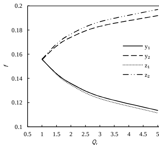
شکل 14 تغییرات ضریب اصطکاک میانگین با Q_r بر روی دیواره‌های مختلف
