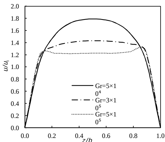
شکل 16 پروفیل سرعت در مقطع x/D_h = 20 برای مقادیر مختلف عدد گراشف در شرایط \phi = 1.5\% و Q_r = 1.5 ، Re = 700 ، AR = 0.5
