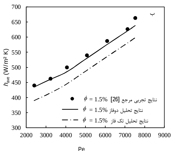
شکل 5 مقایسه نتایج حل عددی با نتایج آزمایشگاهی ناسن و همکاران [26] برای جابجایی اجباری در کانال مربعی در (الف) \phi = 0.5\% و (ب) \phi = 1.5\%
