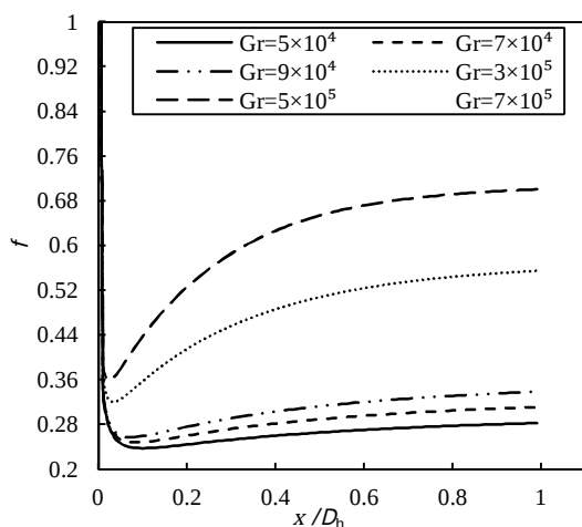
شکل 17 تغییرات ضریب اصطکاک در طول کانال برای مقادیر مختلف عدد گراشف در شرایط \phi = 1.5\% و Q_r = 1.5 ، Re = 700 ، AR = 0.5
