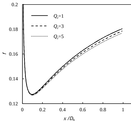
شکل 11 تغییرات ضریب اصطکاک در طول کانال برای مقادیر مختلف نسبت Q_f برای
