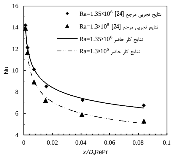
شکل 3 مقایسه نتایج حل عددی با نتایج آزمایشگاهی مارکوس و همکاران [24] در Re = 500 و برای دو عدد رایلی مختلف AR = 0.375
