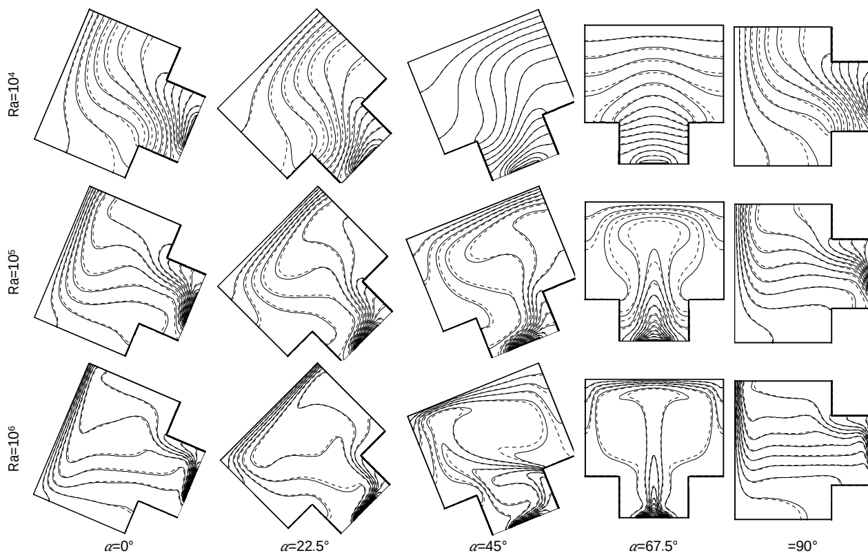
شکل 10 خطوط همدم در زاویه چرخش و ریلی های مختلف در Ha=0 برای سیال خالص (—) و نانوسیال \phi=0.04 (---).
