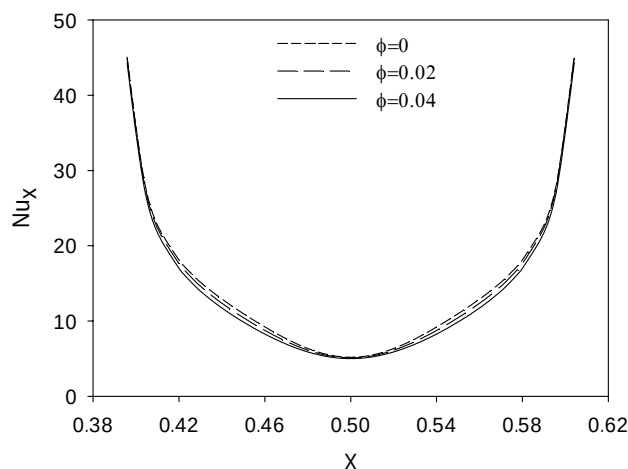
شکل 8 اثر تغییر کسر حجمی نانوذرات مختلف بر نوسلت موضعی ( Ra=10^6, Ha=40 )
