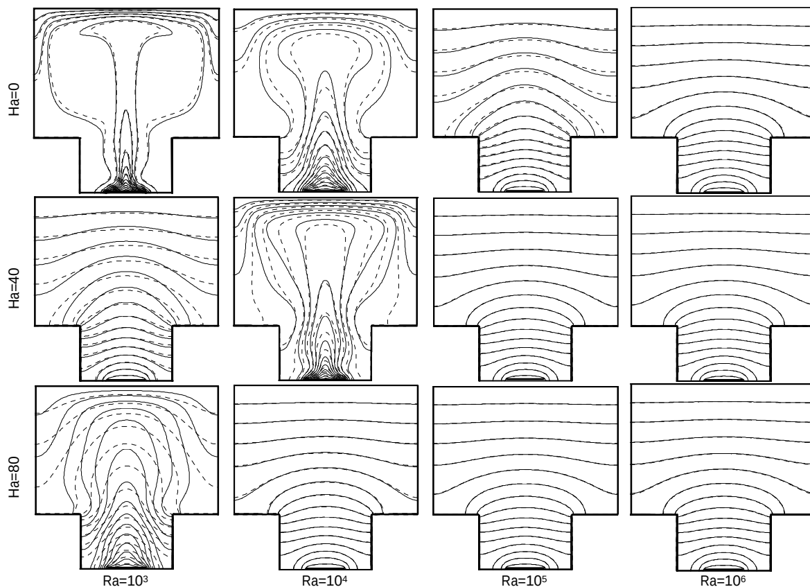
شکل 5 خطوط همدمای در ریلی ها و هارتمن های مختلف برای سیال خالص (—) و نانوسیال \phi=0.04 (---)
