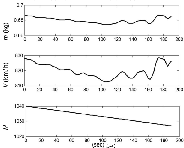
شکل 11 تغییرات عدد ماخ، سرعت و وزن پرنده
