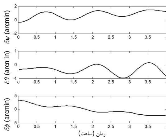
شکل 7 تغییرات خطای وضعیتهای زاویه‌ای برحسب زمان
