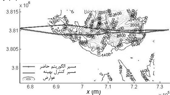
شکل 16 مقایسه مسیرهای منتهج به روش‌های کنترل بهینه و شبکه جریان در شرایط یکسان
