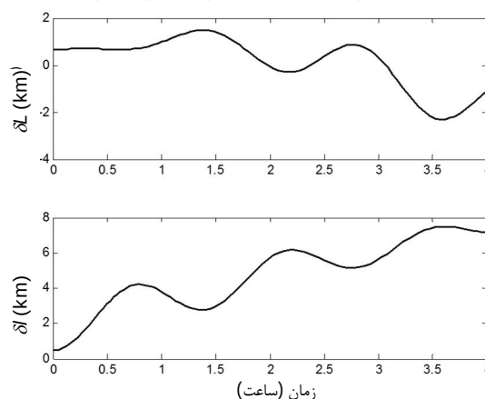
شکل 8 تغییرات خطای موقعیت در دو جهت عرض و طول جغرافیایی برحسب زمان
