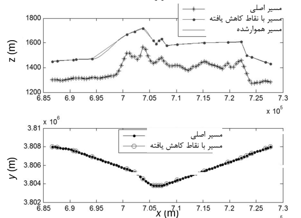
شکل 10 تصویر مسیر در صفحات x-y و x-z و هموار شده آن
