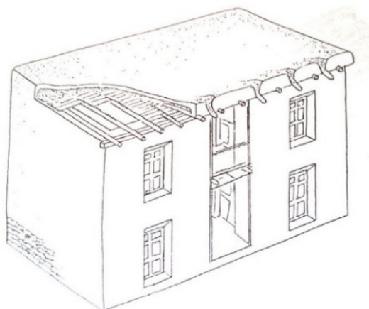
شکل ۴: نمونه رایج خانه‌های مراتع حوزه‌ی کوهستانی «دیوار سنگی یا خشتی، سقف صاف تیرچه پوش» [۴]
