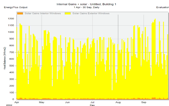
شکل ۱۶: ریتم سیرکولاسیون جذب انرژی خورشیدی در فصل زمستان
