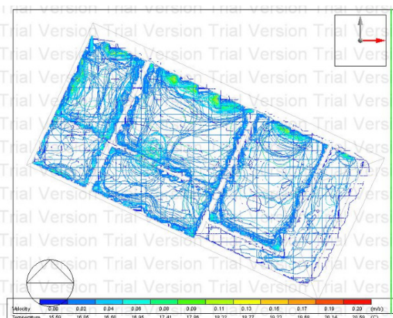
شکل ۱۳: نمودار جریان هوای ساختمان در فصل تابستان
