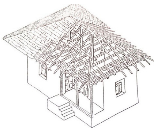
شکل ۵: نمونه‌ی رایج خانه‌های واقع در حوزه‌ی ساحلی «دیوار گلی یا آجری، سقف شیبدار سقال» [۴]
