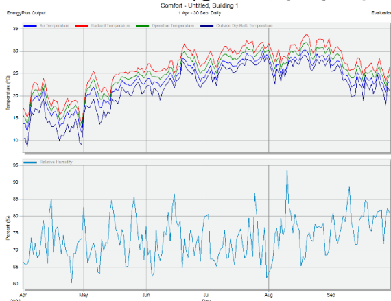
شکل ۱۱: مقایسه دمای ساختمان در مقایسه با دمای بیرون (خط آبی تیره نمودار دمای خارج ساختمان) در فصل تابستان
