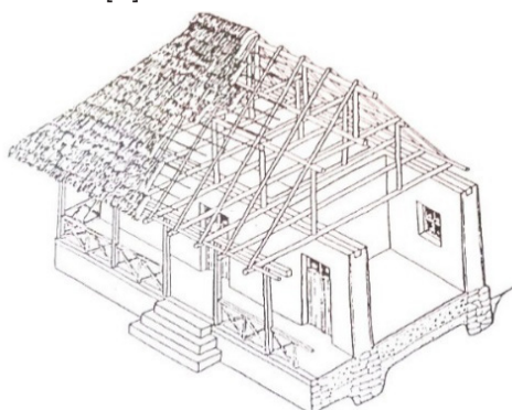
شکل ۳: نمونه‌ی رایج خانه‌های گالی پوش [۴]
