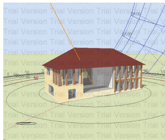
شکل ۱۲: شبیه سازی مدل سه بعدی ساختمان
