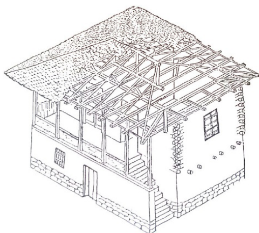
شکل ۲: نمونه‌ی رایج خانه‌های حوزه‌ی کوهپایه‌ای [۴]
