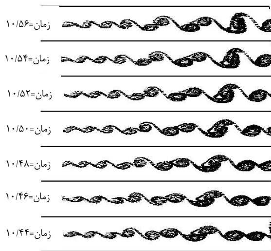
شکل ۵ بردارهای سرعت و موقعیت لحظه‌ای المان‌های گردابه‌ای برای لایه‌برشی با تحریک اجباری برای \mathcal{E}_s = 0 ، \mathcal{E}_f = 0.01\mathcal{M}^* ، نسبت سرعت R = 3 و تعداد ۵ لایه با طول دامنه محاسباتی ۶ در زمانهای مختلف
