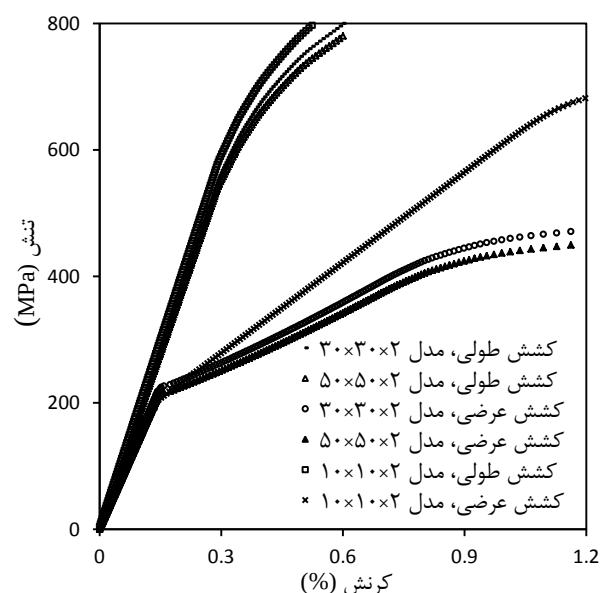
شکل ۸ تأثیر تعداد سلول‌های المان حجمی بر پاسخ تنش-کرنش طولی و عرضی ماده مرکب الیاف کوتاه
