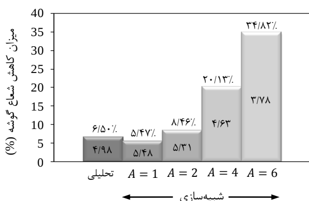
شکل ۹ درصد کاهش شعاع نسبت به حالت کلاسیک در هیدروفرمینگ آلتراسونیک ( P = 60 MPa و F = 20 kHz)
