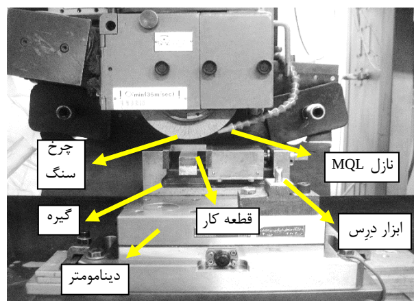
شکل ۳ چیدمان تجهیزات مورد استفاده در انجام آزمایش ها
