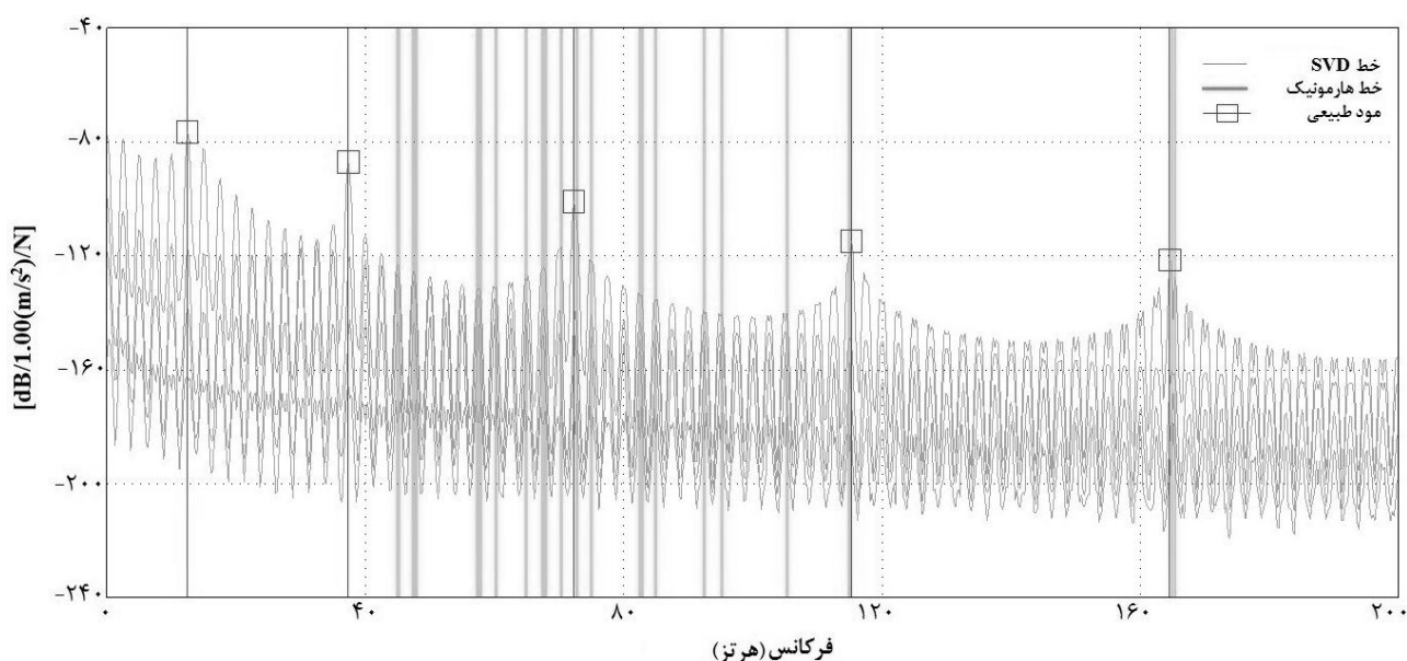
شکل ۴ نمودار طیف مقادیر تکین چگالی توان پاسخ
