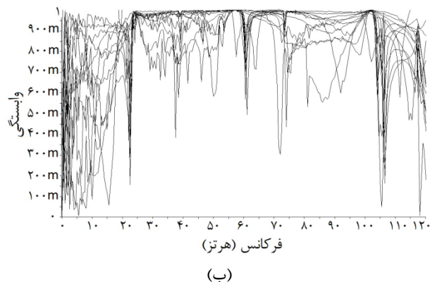
شکل ۹ توابع به دست آمده از آزمایش مودال کلاسیک، (الف) توابع پاسخ فرکانسی (H1)، (ب) توابع وابستگی
