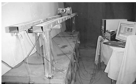
شکل ۱۰ پل تحت آزمایش مودال محیطی (مرحله چهارم آزمایش)
