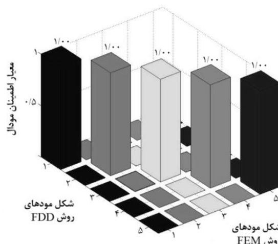
شکل ۶ مقایسه شکل مودهای محاسبه‌شده به روش FEM و FDD با استفاده از معیار MAC
