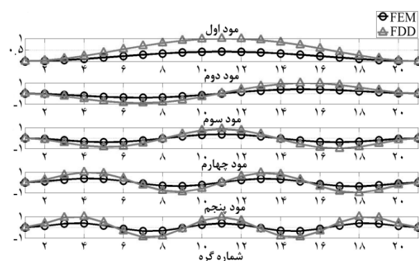
شکل ۵ مودهای به دست آمده از اجزای محدود و روش FDD
