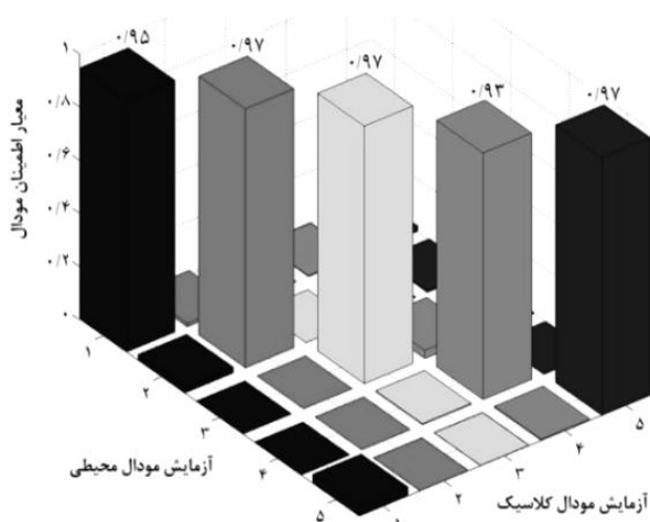
شکل ۱۴ معیار MAC بین شکل مدهای حاصل از آزمایش مودال کلاسیک و آزمایش مودال محیطی
