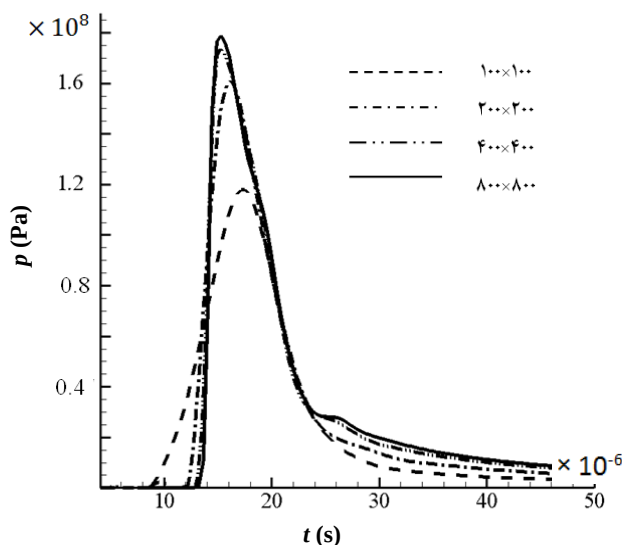
شکل ۳ تاریخچه زمانی تغییرات فشار در موقعیت مکانی (0/175m, 0/875m) به‌ازای تعداد شبکه مختلف
