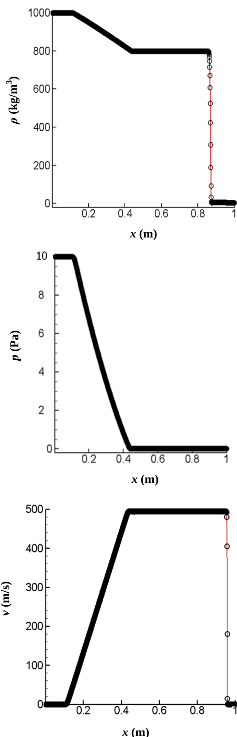
شکل ۲ لوله ضربه گاز-مایع، مقایسه نتایج عددی (نشانه) با نتایج حل دقیق [۹] (خط توپر) و تعداد شبکه ۱۰۰۰ (از بالا به پایین: چگالی مخلوط دوفازی، فشار و سرعت)
