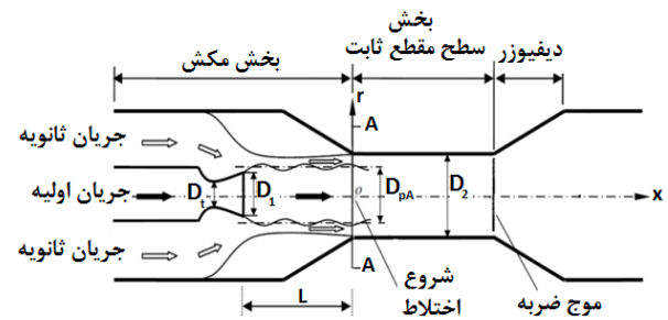
شکل ۴ نمای شماتیکی اجکتور و علایم به کار رفته در مدل سازی
