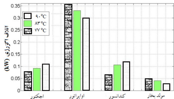
شکل ۱۳ تأثیر دمای مولد بخار بر روی اتلاف انرژی بخش‌های مختلف چرخه در دمای اوپراتور ۱۳/۵ درجه سلسیوس
