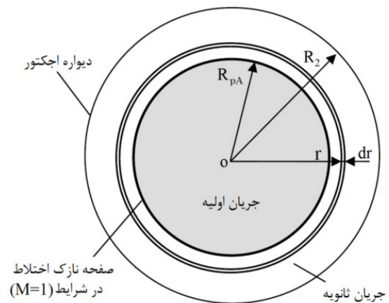
شکل ۶ دیگرام شماتیکی جریان در سطح مؤثر [۹]
