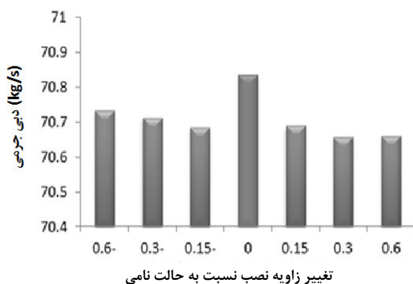
شکل ۳۱ دبی جرمی بر حسب تغییرات نسبت به هندسه نامی
