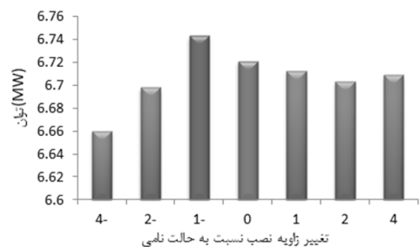
شکل ۲۸ توان بر حسب تغییرات نسبت به هندسه نامی
