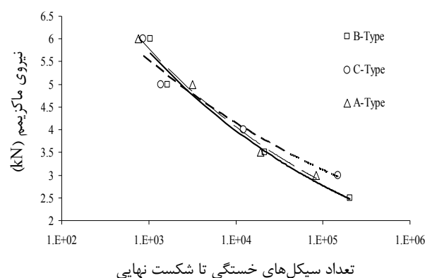
شکل ۲ منحنی تست خستگی اتصالات نقطه‌جوش مورد نظر
