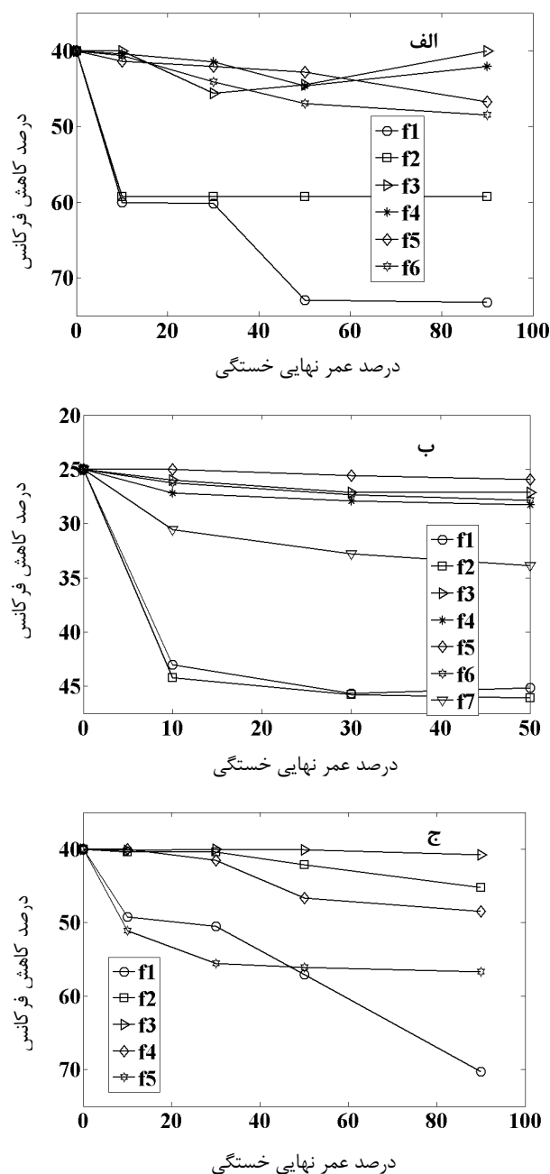
شکل ۱۰ روند تغییرات فرکانس طبیعی اتصالات نوع A، B و C در عمرهای مختلف خستگی. (الف) اتصال A، (ب) اتصال B و (ج) اتصال C
