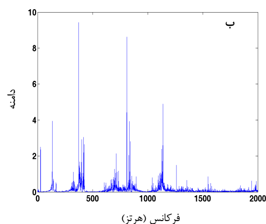
شکل ۹ FRF اتصال نوع A؛ (الف) قبل از اعمال بارگذاری سیکلیک و (ب) بعد از ۱۰ درصد عمر خستگی نهایی
