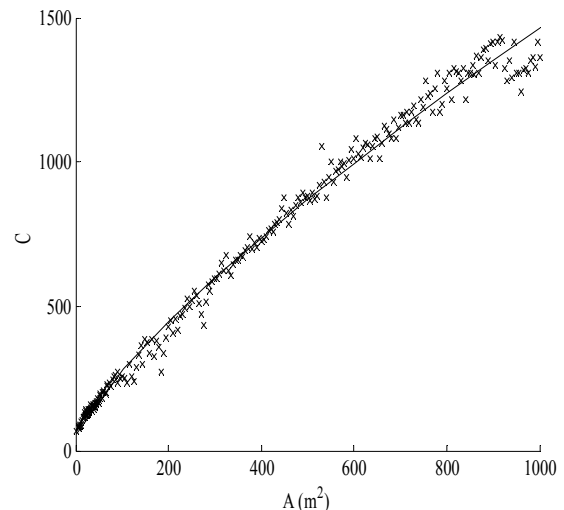
شکل ۳ نحوه برازش داده‌ها برای ساختار کربن استیل در محدوده بیشینه فشار کارکرد بین ۱/۲ تا ۱۰ بار
