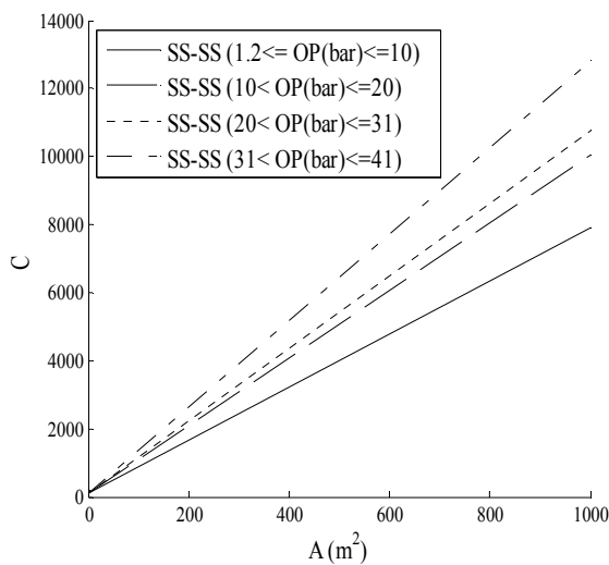
شکل ۴ نمودار روابط تعیین قیمت برای ساختار استیل ضد زنگ ۳۱۶ در محدوده بیشینه فشار کارکرد ۱/۲ تا ۴۱ بار
