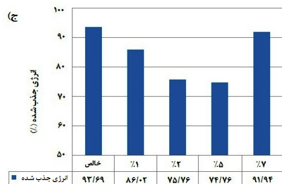
شکل ۴ درصد جذب انرژی اولیه برخورد بر حسب درصد نانورس؛ (الف) سرعت برخورد V_i=130\text{m/s} ، (ب) سرعت برخورد V_i=142\text{m/s} ، (ج) سرعت برخورد V_i=155\text{m/s}
