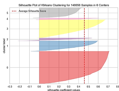
شکل ۴. نمودار Silhouette برای K= ۶
