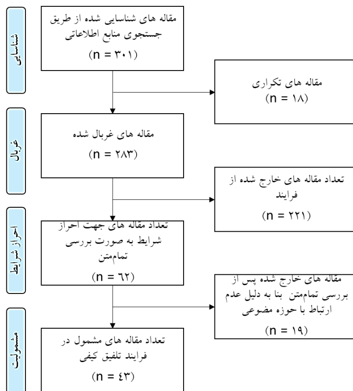
نمودار ۱. فلوچارت فرایند انتخاب مقاله‌های مورد بررسی در مطالعه بر مبنای روش PRISMA
