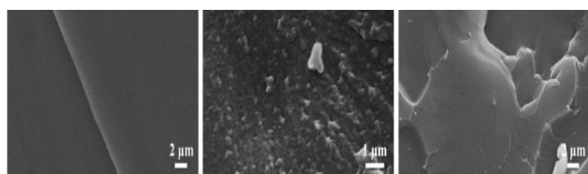
شکل ۱ از چپ به راست رزین اپوکسی، نانوکامپوزیت اپوکسی و نانوکامپوزیت اپوکسی اصلاح‌شده [۱۴]
