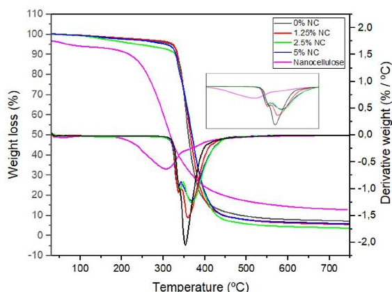
شکل ۳ آزمون گرم‌اوزن‌سنجی رزین اپوکسی و نانوکامپوزیت‌های اپوکسی [۴۷] Figure 3 Thermogravimetric analysis of epoxy resin and epoxy nanocomposites [47]
