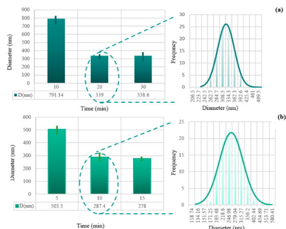
شکل ۲ تعیین اندازه ذرات آهن پیروفسفات میکرونیزه شده به روش (الف) فراصوت و (ب) همگن‌ساز دور بالا
