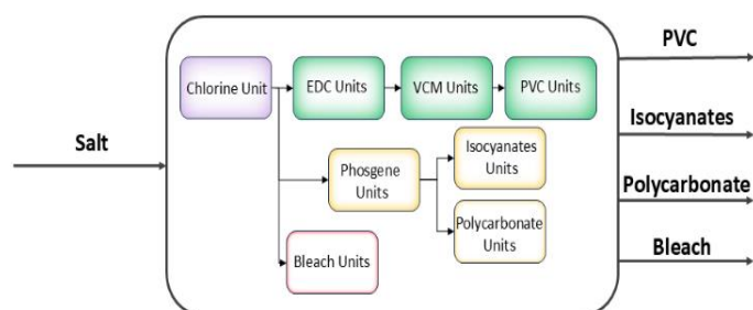
شکل ۴ طرح‌واره نحوه مصرف کلر در صنعت پتروشیمی ایران
