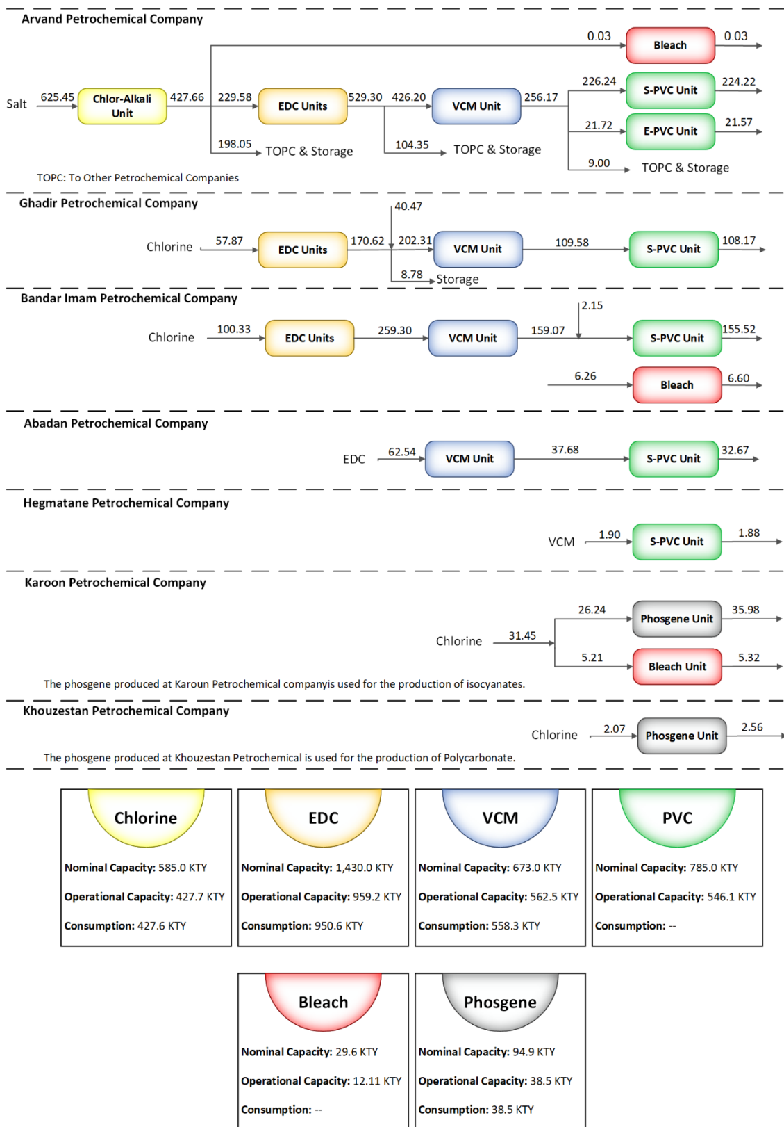
شکل ۵ جریان‌های ورودی و خروجی واحدهای فرایندی که تولیدکننده مواد کلردار هستند Figure 5 Input and output flows of process units producing chlorinated compounds
