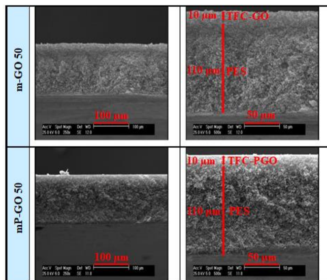
شکل ۸ آزمون SEM مقطعی و اندازه‌گیری ضخامت (با استفاده از ImageJ)
