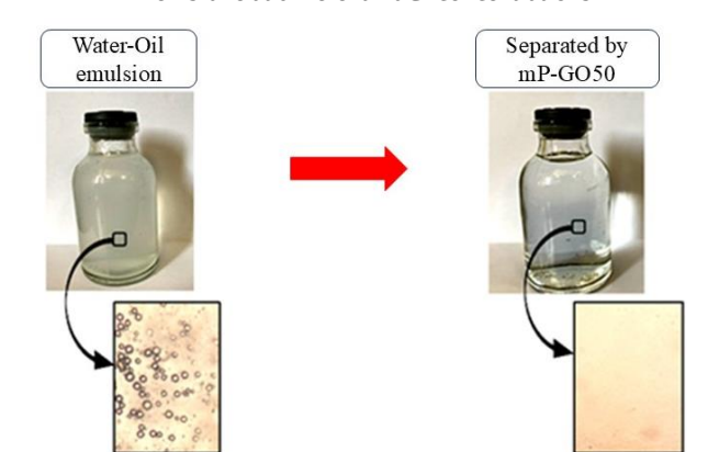
شکل ۵ عکس دیجیتالی و عکس میکروسکوپ نوری از امولسیون آب-روغن جداسازی شده توسط غشای mP-GO50
