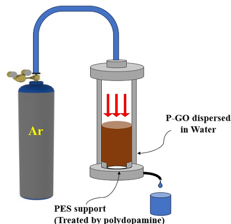
شکل ۱ طرح‌واره روش خودآرایی به کمک فشار که برای ساخت غشاهای لایه‌ای mP-GO به کار می‌رود
