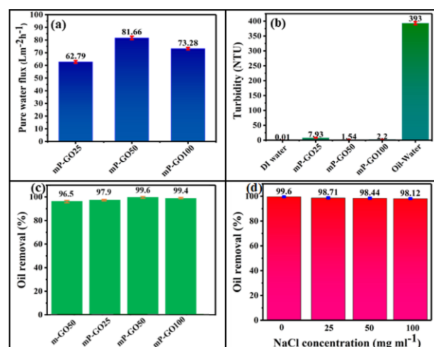
شکل ۴ (الف) شار آب خالص، (ب) کدورت امولسیون اولیه و محلول‌های عبوری از غشا و (ج) درصد حذف روغن غشاهای لایه‌ای بر پایه‌ی GO-50 و P-GO. (د) مقایسه‌ی بازده حذف روغن غشای mP-GO50 در غلظت‌های مختلف نمک NaCl
