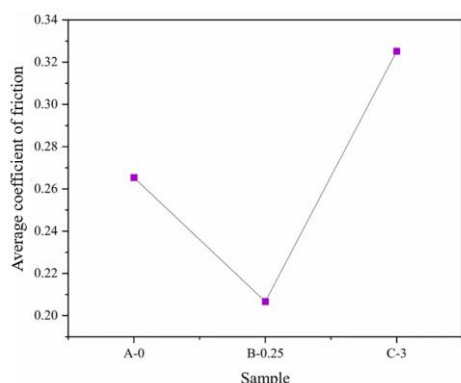
شکل ۴ میانگین ضریب سایش نمونه‌ها Figure 4 Average coefficient of friction of the samples
