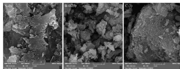
شکل ۳ تصاویر FESEM نمونه بنتونیت (A-0) بنتونیت خام، (B-0.25) بنتونیت فعال‌سازی شده با اسید ۰/۲۵ مولار، (C-3) بنتونیت فعال‌سازی شده با اسید ۳ مولار Figure 3 FESEM images of bentonite samples: A-0) Raw bentonite, B-0.25) Acid-activated bentonite with 0.25 M acid, C-3) Acid-activated bentonite with 3 M acid
