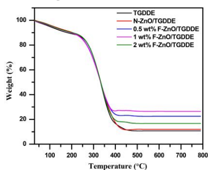
شکل ۴ نمودار گرمایزنی رزین اپوکسی و نانوکامپوزیت‌های اپوکسی [۵۲] Figure 4 Thermogravimetric analysis (TGA) curves of epoxy resin and epoxy nanocomposites [52]
