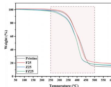
شکل ۳ نمودار گرمایزنی رزین اپوکسی و نانوکامپوزیت‌های اپوکسی [۴۳] Figure 3 Thermogravimetric analysis (TGA) curve of epoxy resin and epoxy nanocomposites [43]
