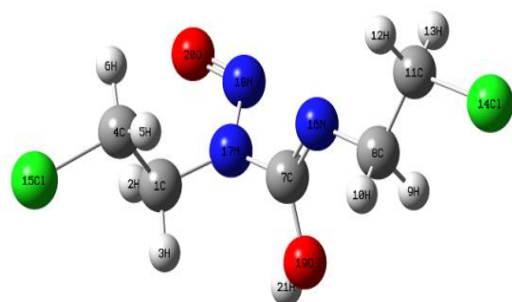
شکل ۲ ساختار بهینه توتومر T1 و T2 با استفاده از Aug-cc-pVDZ
