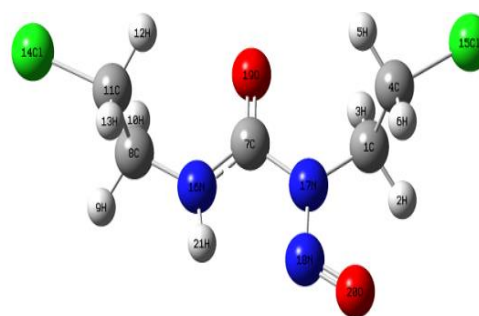
شکل ۲ ساختار بهینه توتومر T1 و T2 با استفاده از Aug-cc-pVDZ
