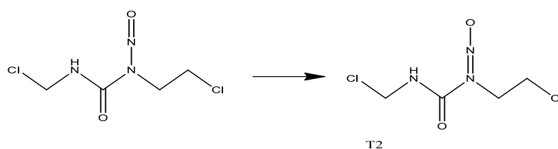
شکل ۱ ساختار کارموستین و توتومرها
