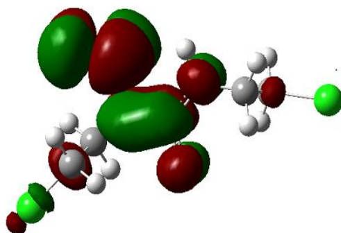
شکل ۴ طرح HOMO-LUMO کارموستین با استفاده از Aug-cc-pVDZ
