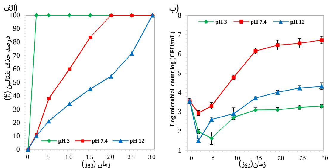
شکل 4 بررسی اثر pH اولیه بر عملکرد \text{CaO}_2 در آب زیر زمینی، الف - درصد حذف نفتالین در نمونه‌ها، ب - تغییرات جمعیت میکروبی در نمونه‌های آب زیرزمینی
