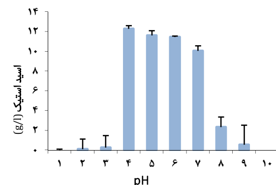
نمودار ۲) اثر pH بر میزان تولید استیک‌اسید توسط Acetobacter sp. 10 محیط کشت‌های EYB (۵۰ میلی‌لیتر در فلاسک‌های ۲۵۰ میلی‌لیتری) از طریق افزودن هیدروکلریک‌اسید (HCl) و سدیم‌هیدروکسید (NaOH) تنظیم شد. دمای ۳۰°C به مدت ۲۴ ساعت
