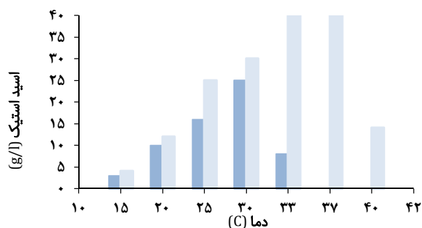
نمودار ۸ مقایسه تحمل دمایی دو سویه گرمپای و مزوفیل. سویه مزوفیل سویه گرمپای Acetobacter sp. A10 . با لحاظ شرایط بهینه pH برابر ۴ و هوادهی با سرعت ۱۵۰ دور در دقیقه در ارلن‌های شیاردار حاوی محیط‌های کشت EYB (۵۰ میلی‌لیتر در فلاسک‌های ۲۵۰ میلی‌لیتری) در مدت ۲۴ ساعت
