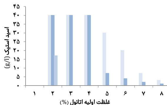
نمودار ۹ اثر غلظت اولیه اتانول بر تولید استیک اسید توسط سویه Acetobacter sp. A10 در ۳ دمای مختلف: ۳۳°C، ۳۷°C و ۴۰°C با رعایت شرایط بهینه. با لحاظ شرایط بهینه pH برابر ۴ و هوادهی با سرعت ۱۵۰ دور در دقیقه در ارلن‌های شیاردار حاوی محیط‌های کشت EYB (۵۰ میلی‌لیتر در فلاسک‌های ۲۵۰ میلی‌لیتری) در مدت ۲۴ ساعت
