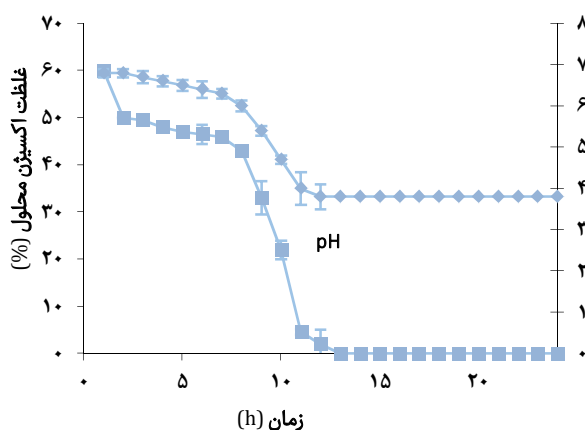
نمودار ۶ تولید استیک اسید توسط سویه Acetobacter sp. A10 براساس تغییرات pH و اکسیژن در شرایط ثابت کشت در یک فرمانتور ۲ لیتری حاوی ۵۰۰ میلی‌لیتر محیط کشت EYB در دمای ۳۳°C به مدت ۲۴ ساعت با غلظت اولیه اتانول ۴٪، سرعت همزن ۲۵۰ دور در دقیقه و حجم اکسیژن ۱۷vvm
