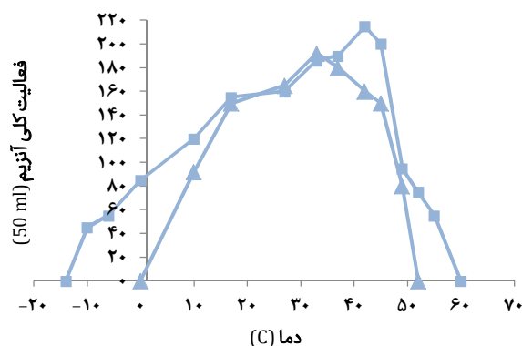
نمودار ۷ فعالیت آنزیمی کل و تحمل حرارتی آنزیم الکل‌دهیدروژناز (ADH) در سویه گرمپای Acetobacter sp. A10 و یک سویه مزوفیل در دماهای مختلف
