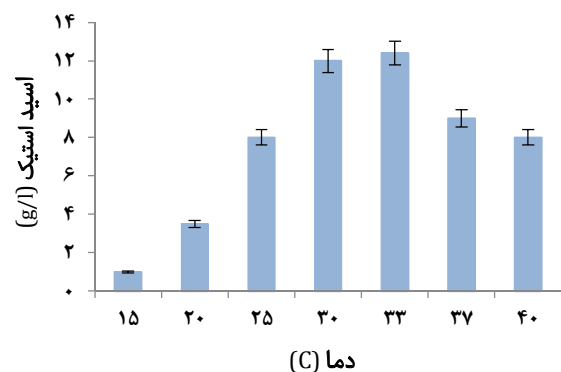
نمودار ۱) اثر دما بر میزان تولید استیک‌اسید توسط سویه Acetobacter sp. 10 در فلاسک‌های ارلن‌مایر ۲۵۰ میلی‌لیتری با ۵۰ میلی‌لیتر محیط کشت EYB در مدت ۲۴ ساعت
