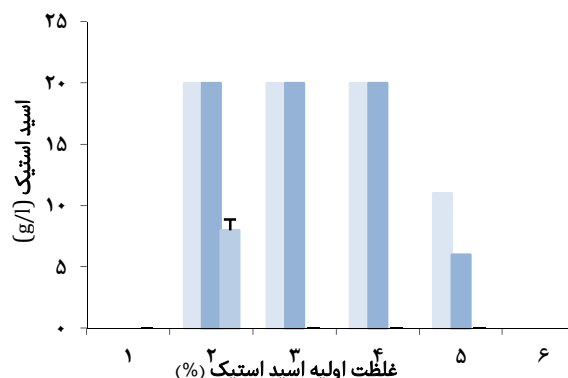
نمودار ۱۰ اثر غلظت اولیه استیک اسید بر تولید استیک اسید توسط سویه Acetobacter sp. A10 در ۳ دمای مختلف: ۳۳°C، ۳۷°C و ۴۰°C به محیط‌های کشت EYB (۵۰ میلی‌لیتر در فلاسک‌های شیاردار ۲۵۰ میلی‌لیتری) به غلظت‌های مختلف استیک اسید افزوده شد. بعد از تلقیح کشت‌ها در ۳ دمای مختلف ۳۳°C، ۳۷°C و ۴۰°C به مدت ۲۴ ساعت با سرعت ۱۵۰ دور در دقیقه گرم‌گذاری شدند
