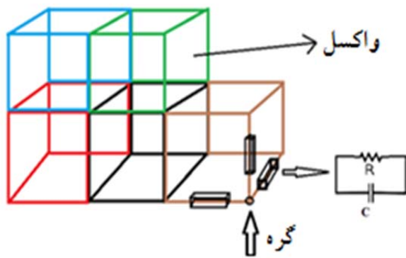
شکل ۳) نمایش واکسل و نحوه اختصاص امپدانس در روش شبکه انتقالی
