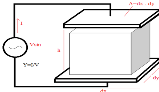
شکل ۵) نمایی از نحوه محاسبه خواص الکتریکی هر لایه و موازی بودن لایه‌های اپیدرم. بلوکی که بین صفحات خازن شبیه‌سازی قرار می‌گیرد شامل مدل‌های (ناهمگن) سلولی با اندامک‌ها است
