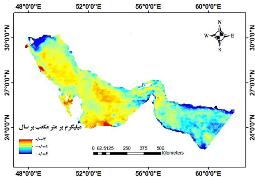
شکل ۵. نقشه سنس استیمیتور غلظت کلروفیل a (میلیگرم بر متر مکعب بر سال) در خلیج فارس و دریای عمان در کل دوره مطالعه
