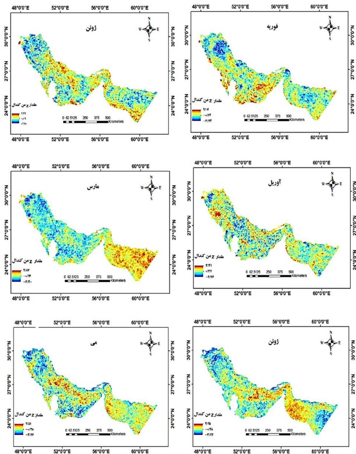
شکل ۹. نقشه تغییرات مکانی مقدار Z من کندانال غلظت کلروفیل a خلیج فارس و دریای عمان در شش ماهه اول سال‌های ۲۰۰۳ تا ۲۰۱۸
