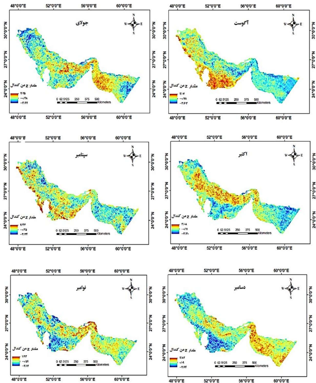
شکل ۱۰. نقشه تغییرات مکانی مقدار Z من کندیال غلظت کلروفیل a خلیج فارس و دریای عمان در شش ماهه دوم سال‌های ۲۰۰۳ تا ۲۰۱۸
