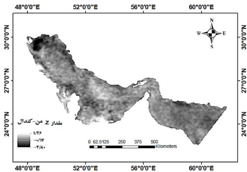
شکل ۶. نقشه تغییرات مکانی مقدار Z من-کنداال غلظت کلروفیل a در خلیج فارس و دریای عمان در کل دوره مطالعه
