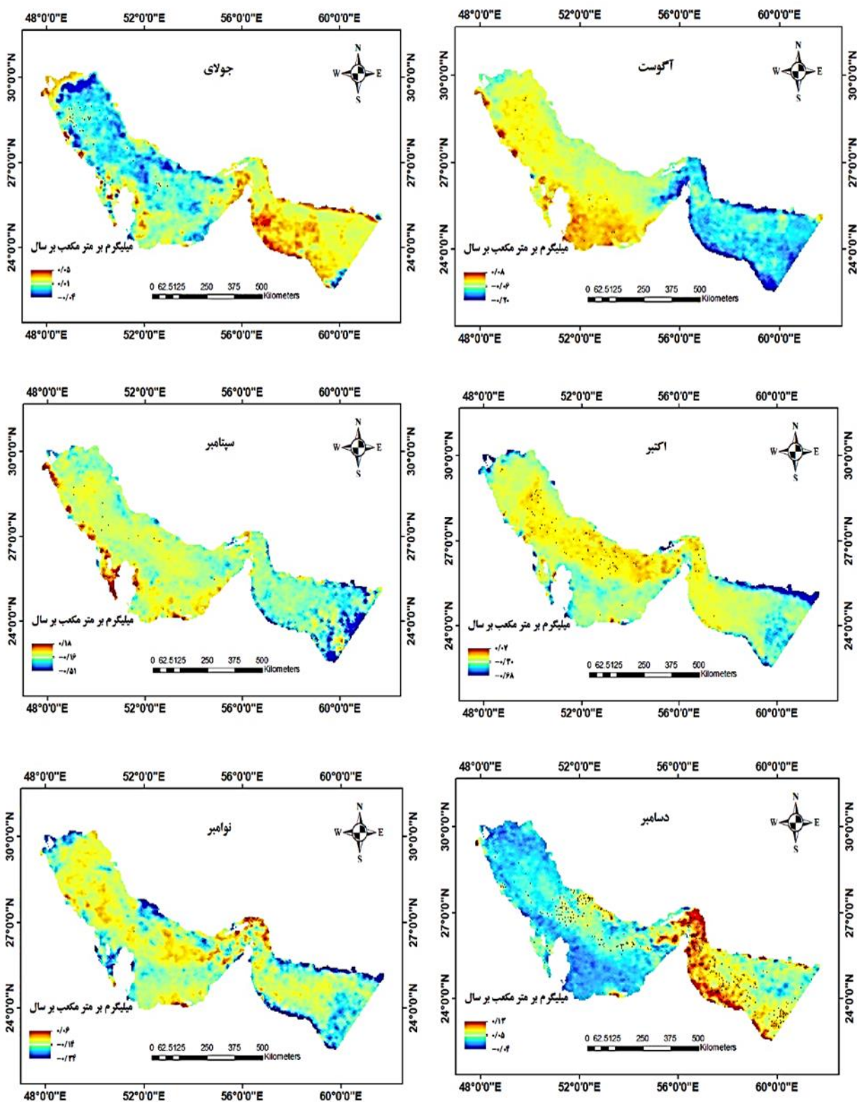
شکل ۸: نقشه سنس استیمیتور ماهانه غلظت کلروفیل a (میلیگرم بر مترمکعب بر سال) خلیج فارس و دریای عمان در شش ماهه دوم سال‌های ۲۰۰۳ تا ۲۰۱۸. نقاط سیاه رنگ نشان دهنده معنی‌داری در سطح پنج درصد ( p < 0.05 )
